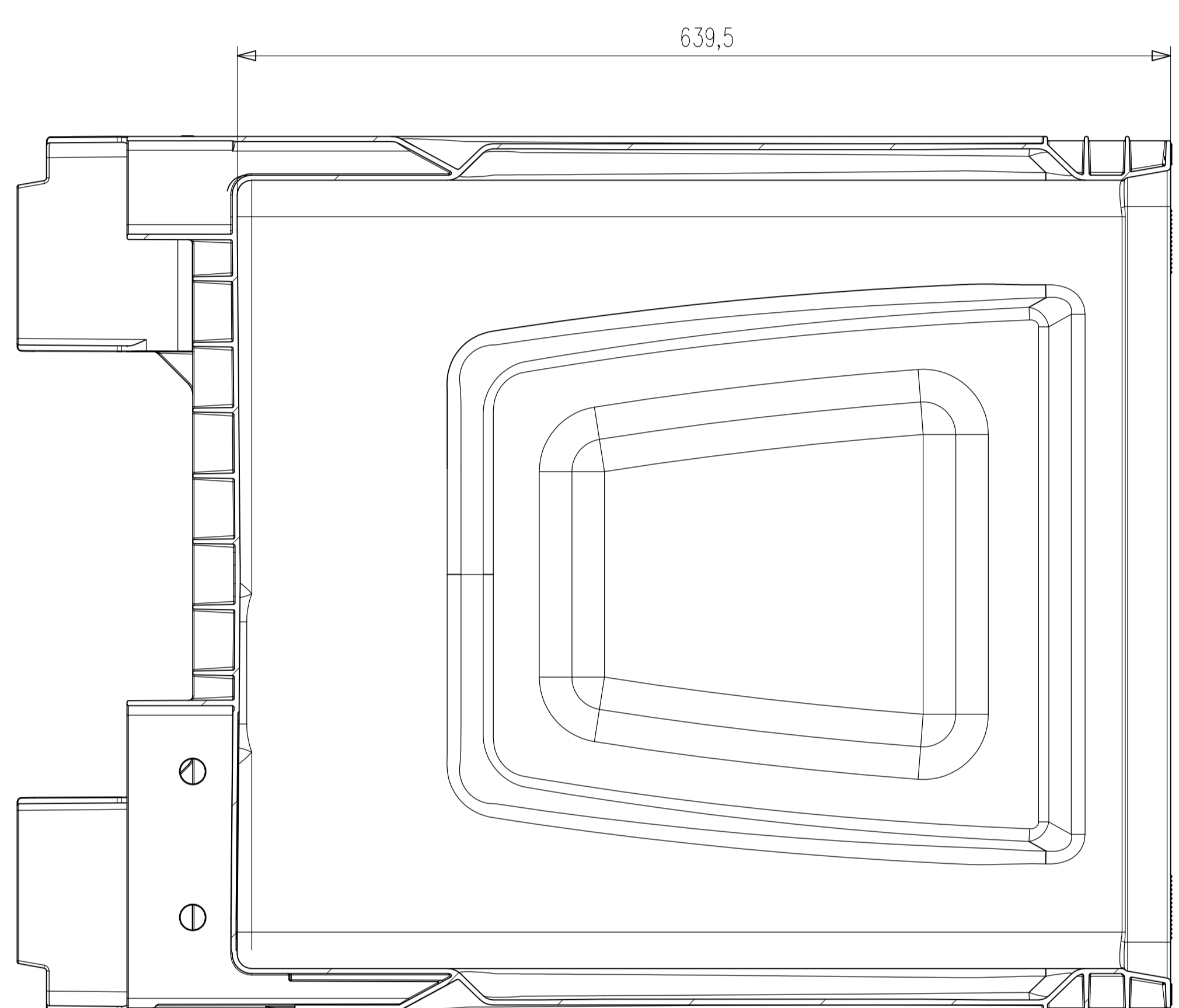
Schnitt A-A
